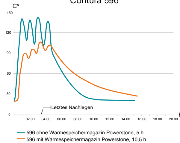
Wärme-Abgabediagramm Contura 596
